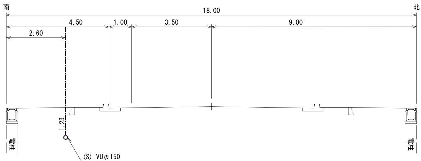
標準断面図
