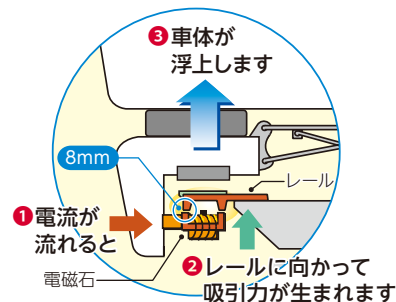
リニモが浮上するしくみ
