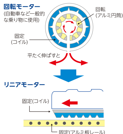
リニモが進むしくみ
