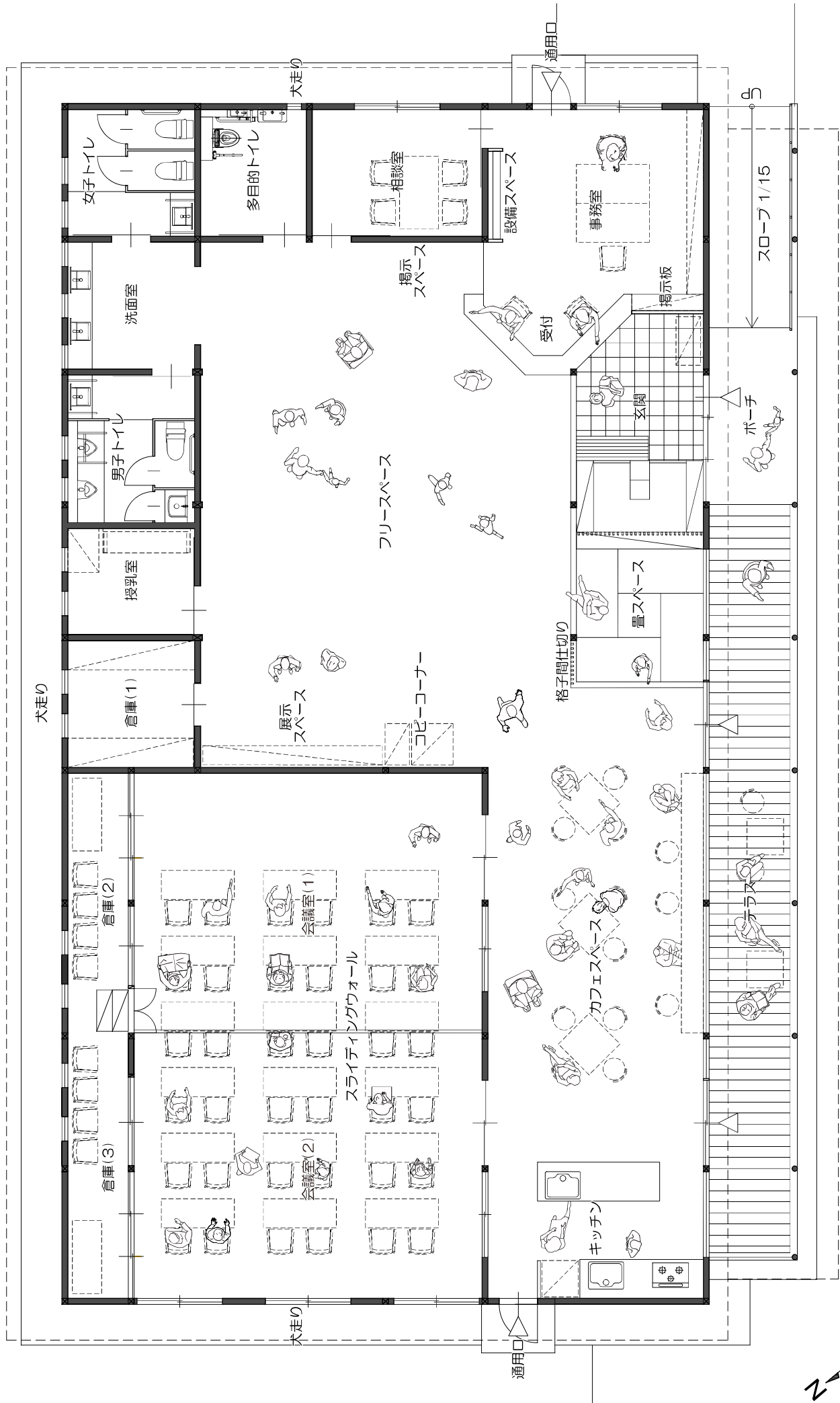
平面図 S=1:100
