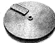
拍子木切り円板一枚刃式
