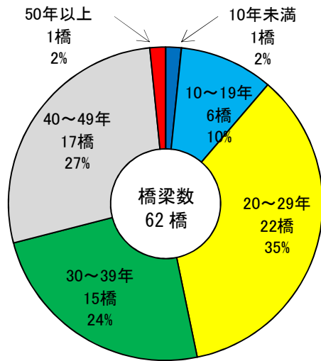
図-3.4 現在の年齢別橋梁割合
