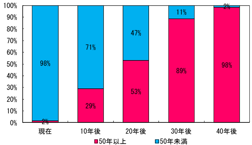
図-3.5 架設後50年以上の橋梁割合推移
