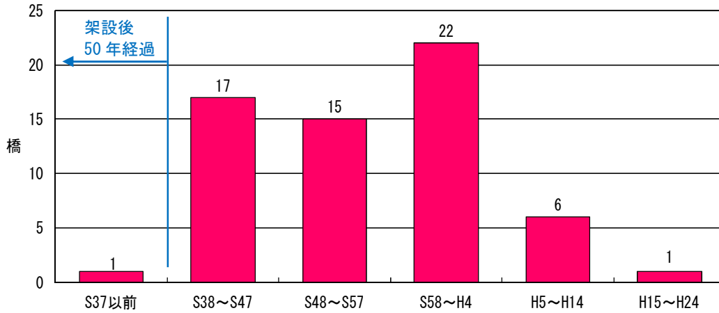
図-3.3 架設年度別の橋梁数
