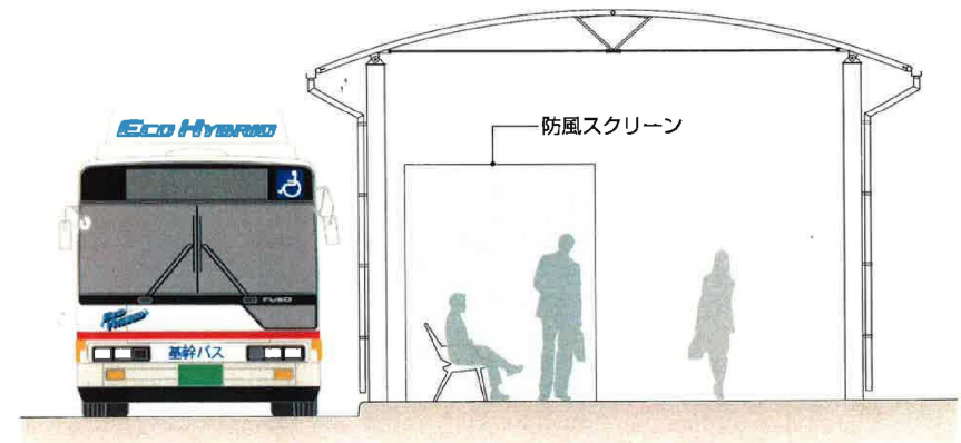
案2：テント屋根断面イメージ
