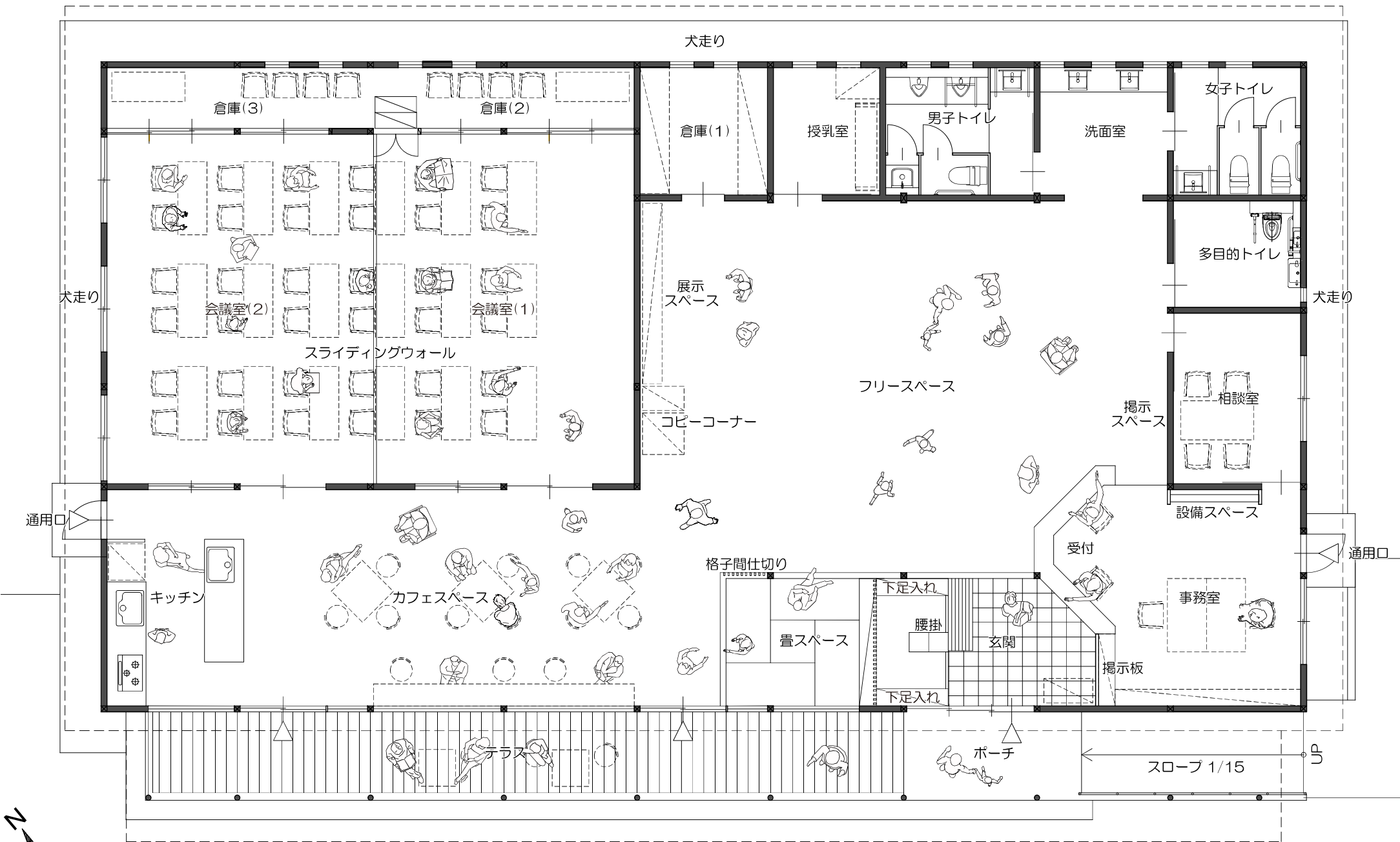
平面図 S=1:100
